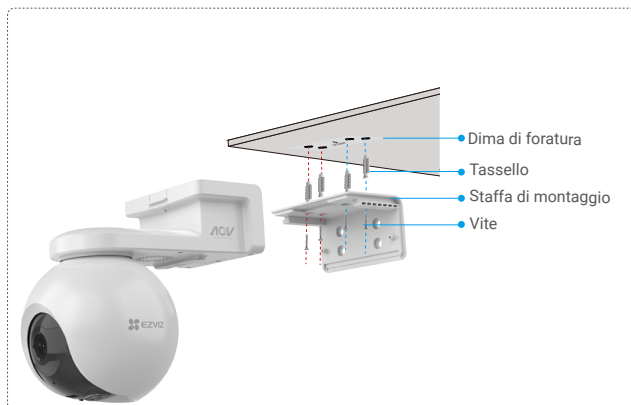
Fig. 1 Montaggio a soffitto
