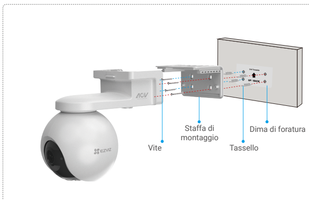
Fig. 2 Montaggio a parete
